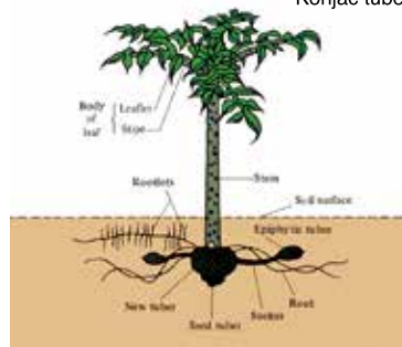
こんにやく植物の模式図 Diagram of Amorphophallus Konjac, K.Koch
